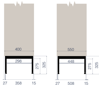
Benram med höjd 325-342 mm
