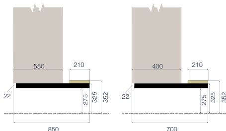
Bänkkonsol med sits av björklaminat
