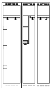
PRO C 100 Skåp 5, 3 och 2
