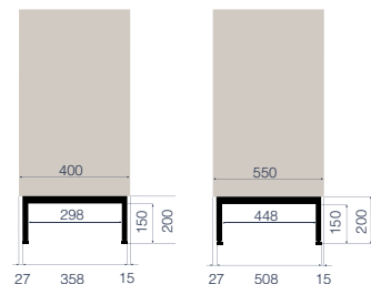
Benram med höjd 200-217 mm
