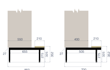
Bänkstativ med sits av björklaminat
