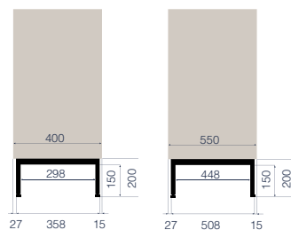
Benram med höjd 200-217 mm
