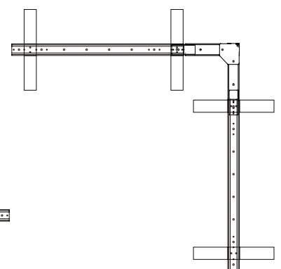
S616 | Hörn för 1 Modul | 1x1 Balk S614 | Singel för 4 Moduler | 2x2 Balkar
